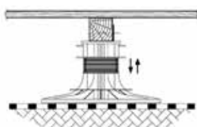
8 platelages (lames + lambourdes) sur plots géotextiles et sol brut stabilisés
